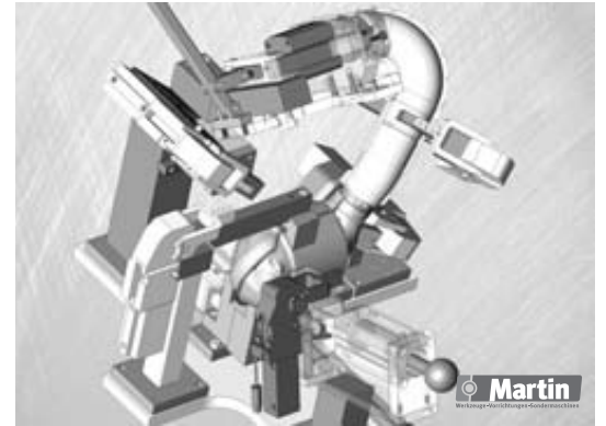
Schweissvorrichtungen für Rohre und Bleche
